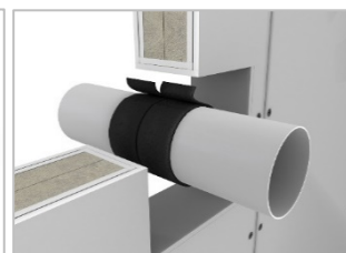
Aanbrengen* aan beide zijden van de brandbare buis vlak met doorvoeringschot
