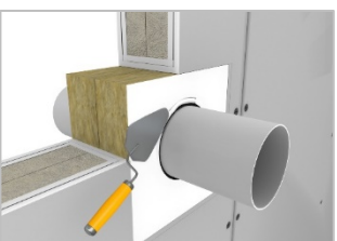
Oppervlak glad afwerken
